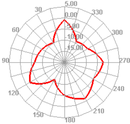
1740.000MHz E1
