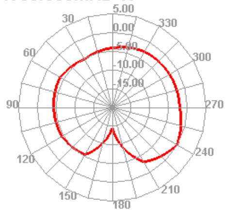
4980.000MHz H
