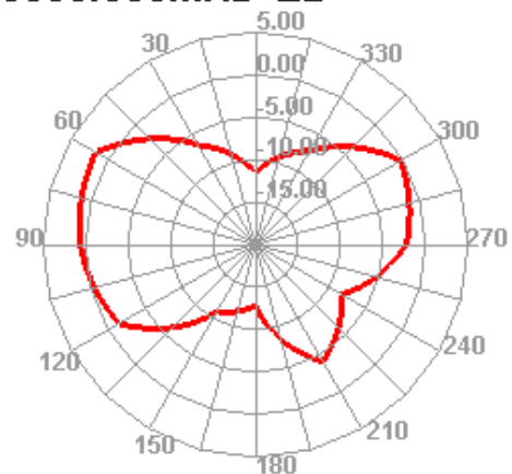
3300.000MHz E2
