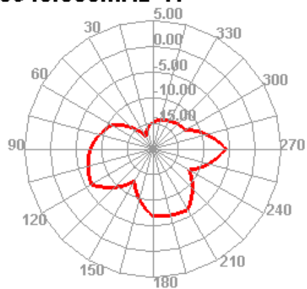
5940.000MHz H
