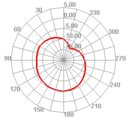
1200.000MHz H
