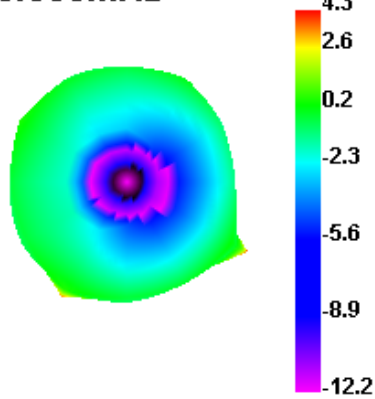
2700.000MHz
