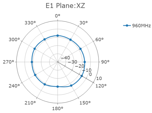
E1-Plane
