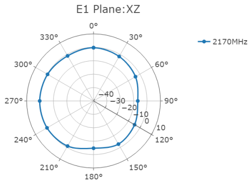
E1-Plane
