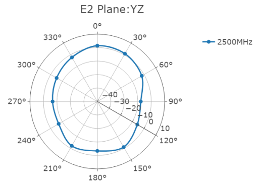
E2-Plane
