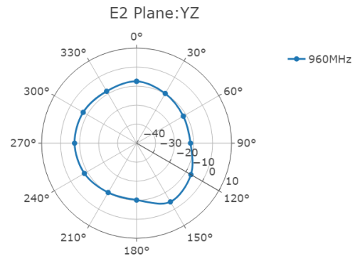
E2-Plane
