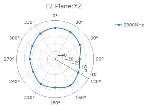
E2-Plane
