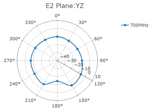
E2-Plane
