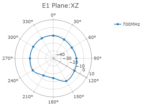
E1-Plane
