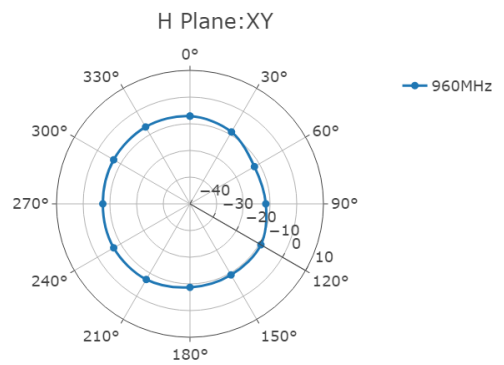
H-Plane
