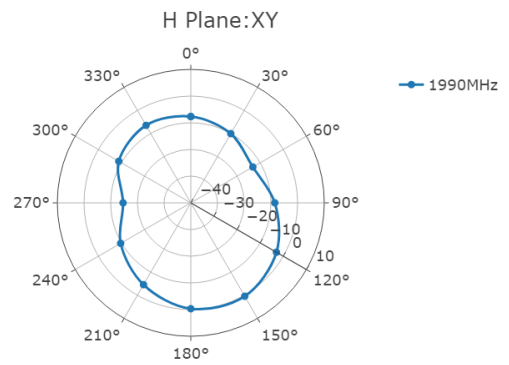
H-Plane
