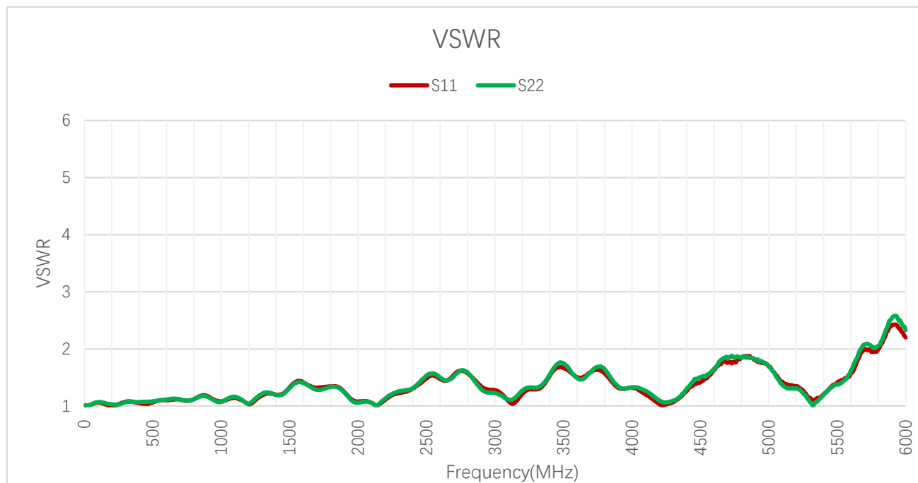
VSWR
