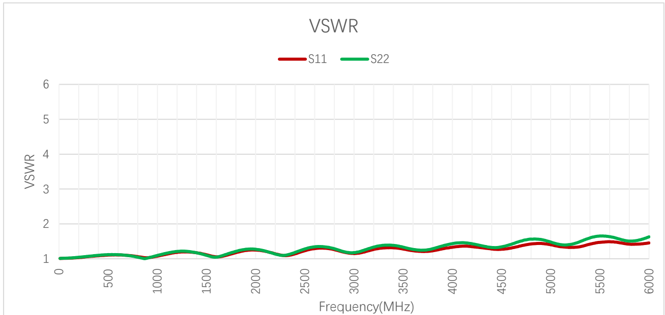
VSWR
