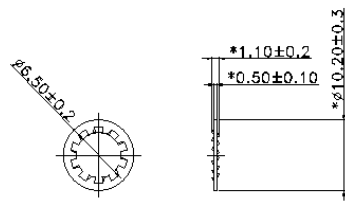
WASHER (ten teeth)
