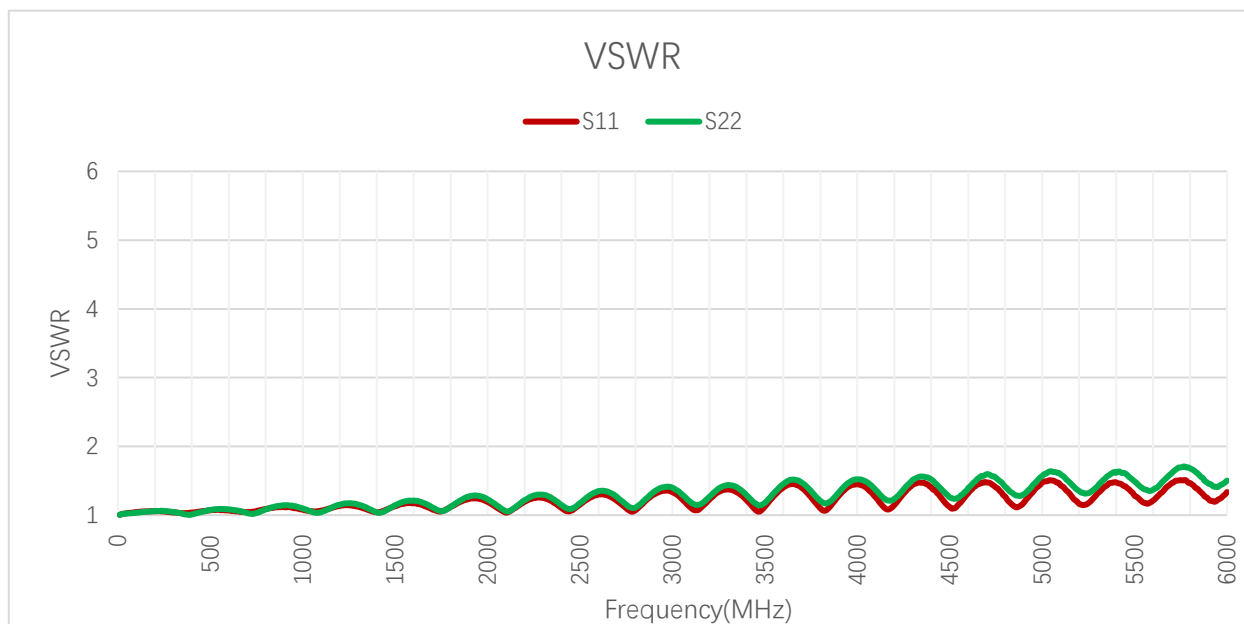
VSWR
