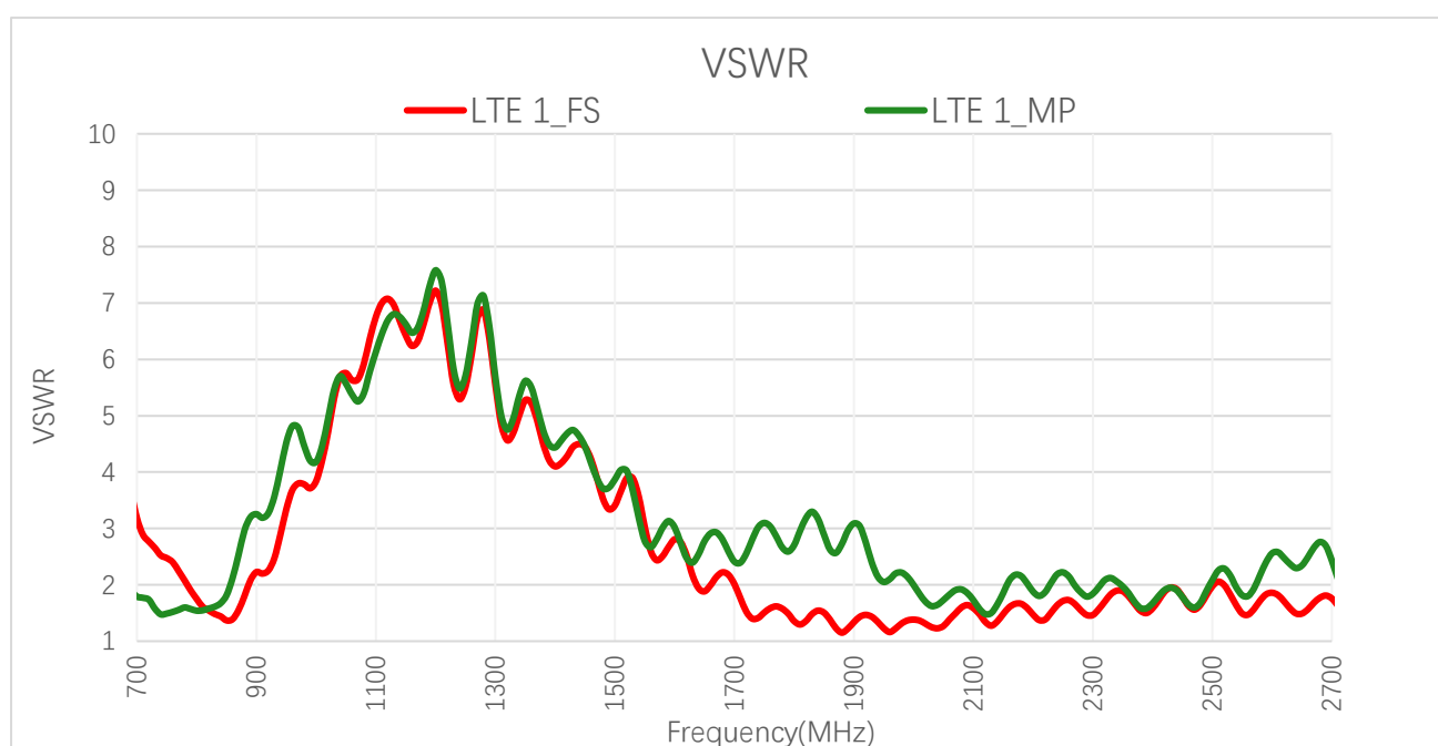
VSWR – LTE 1
