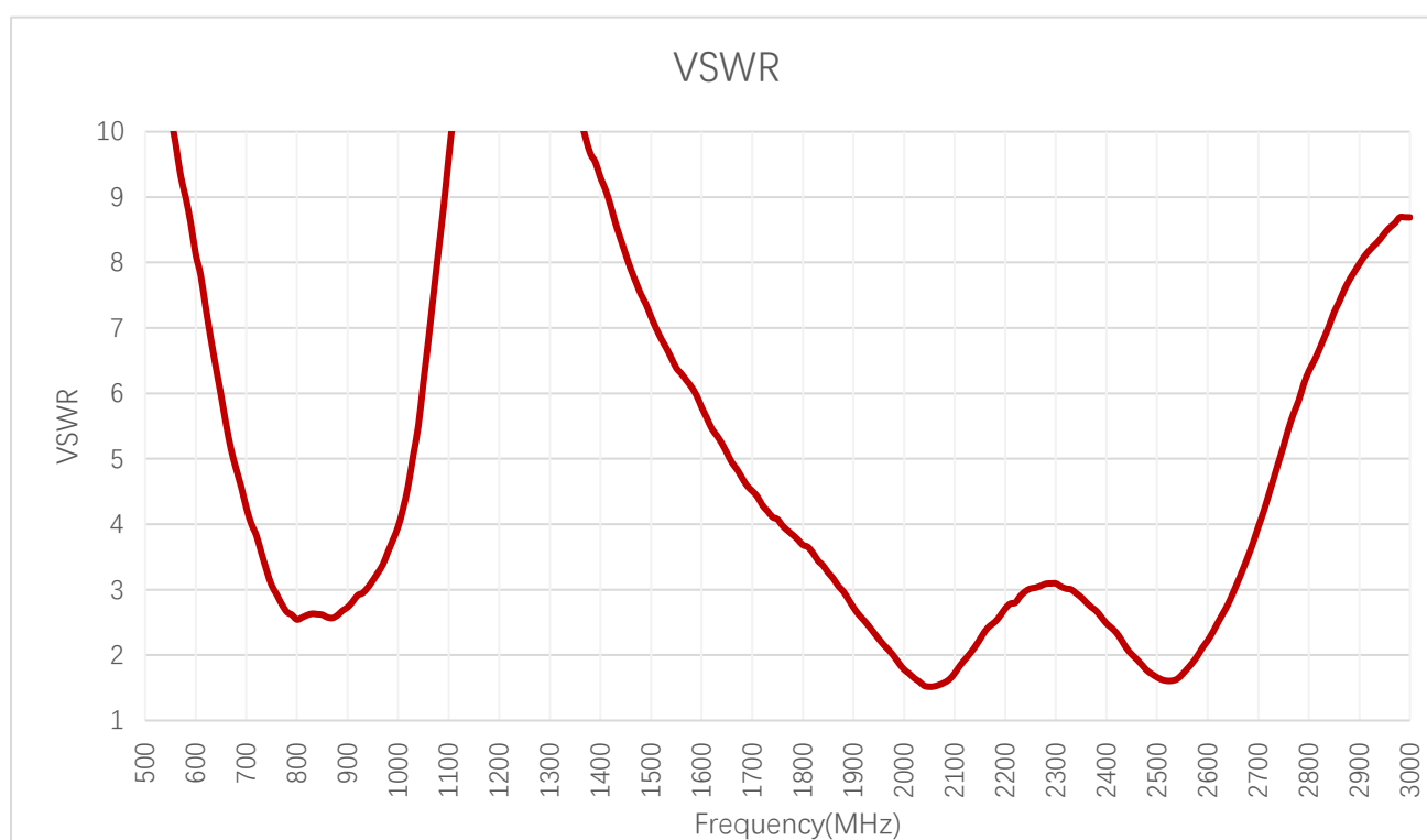
VSWR
