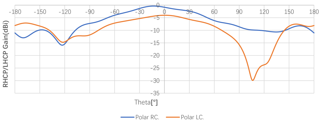
RHCP and LHCP 1575MHz(Phi=0 deg)
