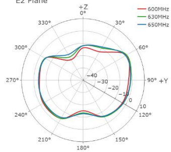
E2 Plane
