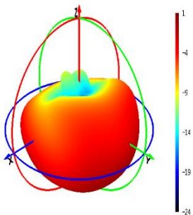
E1 Plane
