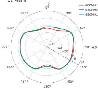
E1 Plane
