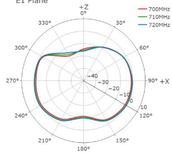
E1 Plane
