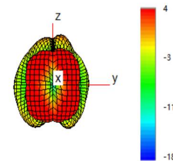
5500 MHz
