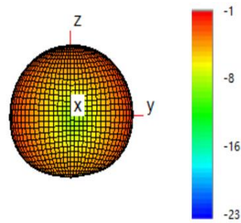
460 MHz
