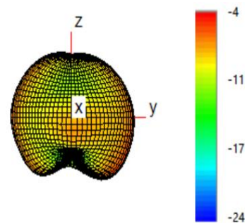
630 MHz
