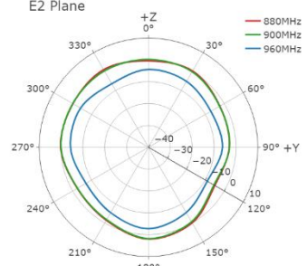
E2 Plane
