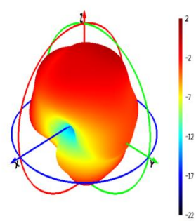
E1 Plane
