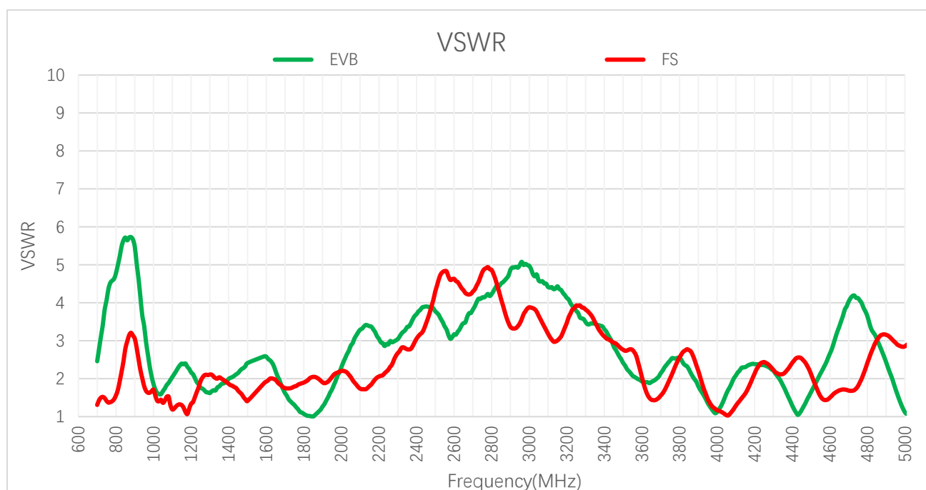
VSWR
