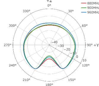
E2 Plane
