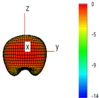
E1 Plane
