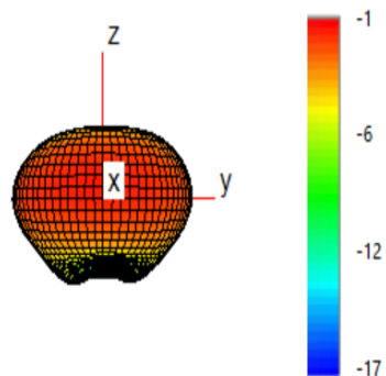
E1 Plane
