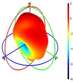
1176 MHz
