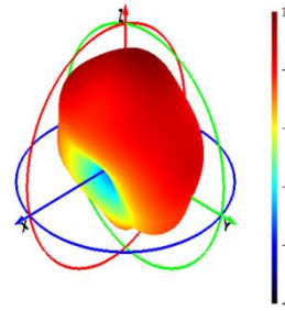
1248 MHz
