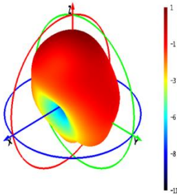
1227 MHz
