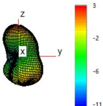
4700 MHz
