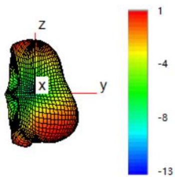
5500 MHz
