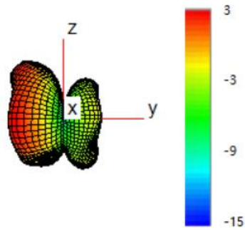
1740MHz
