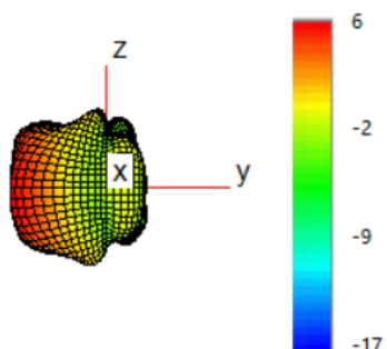
3600 MHz
