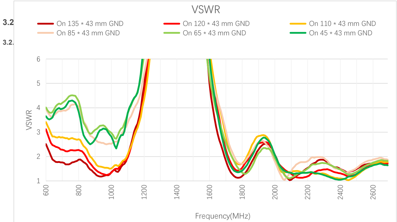
VSWR
