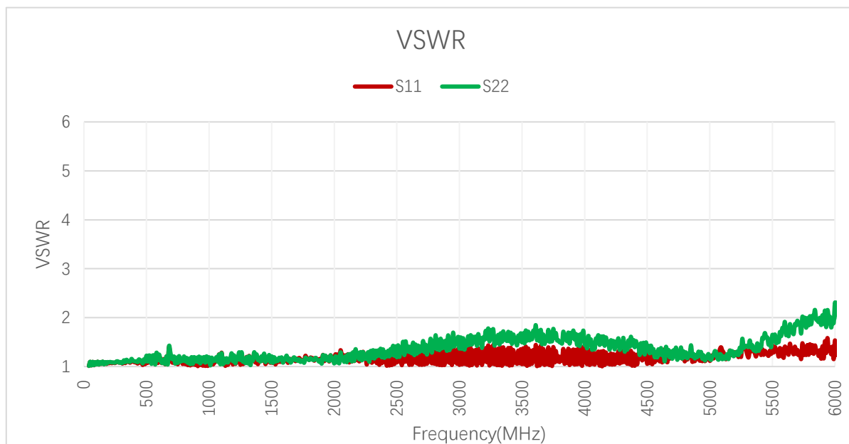
VSWR
