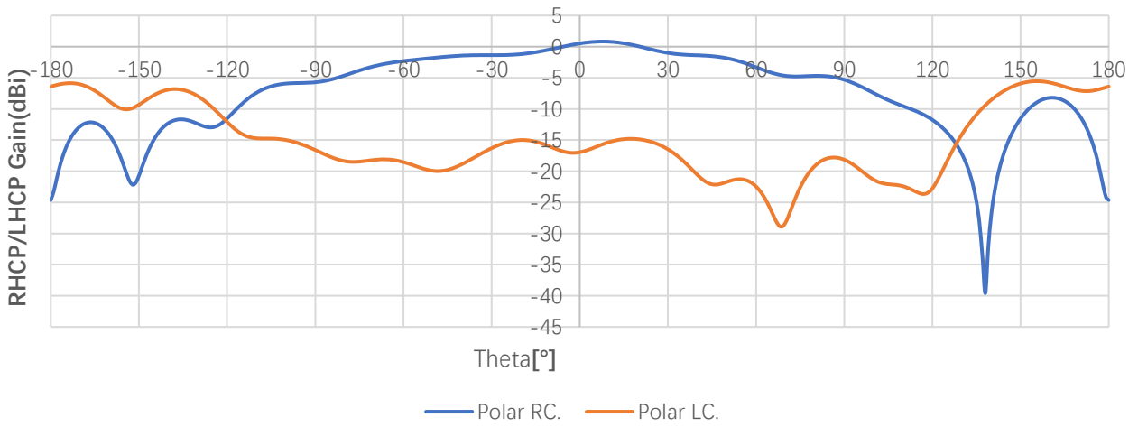
RHCP and LHCP 1561MHz(Phi=90 deg)
