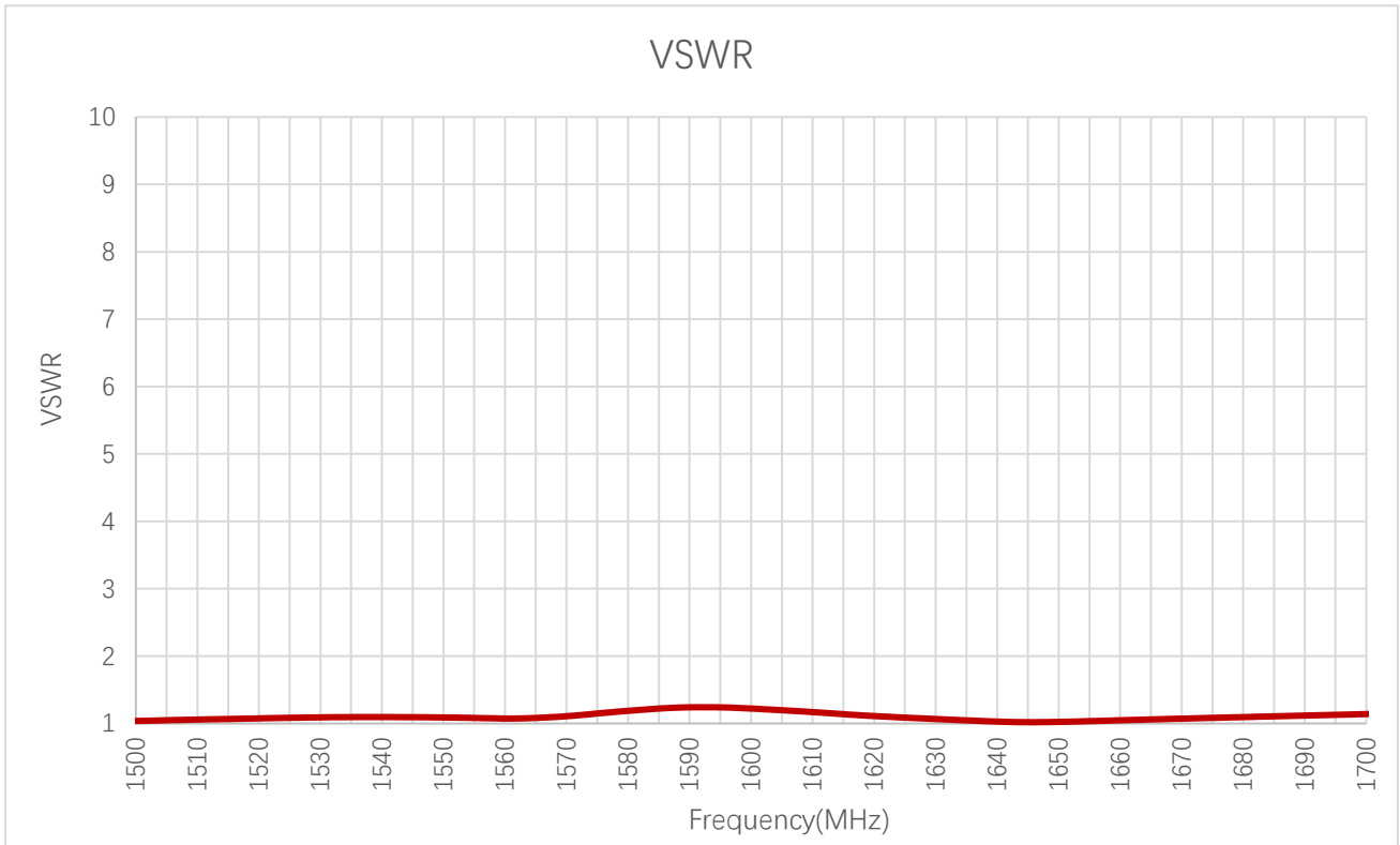
VSWR
