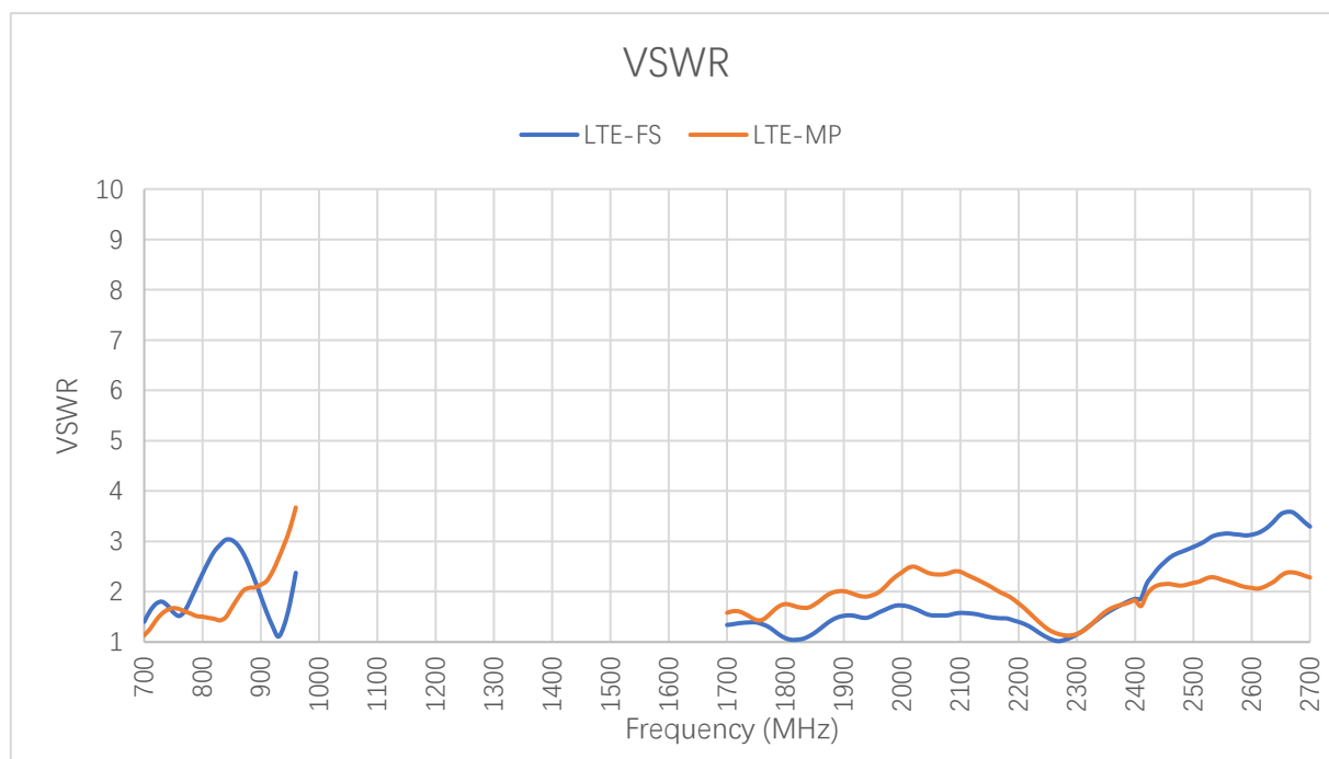
VSWR – LTE
