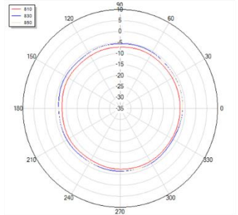
Theta=90
