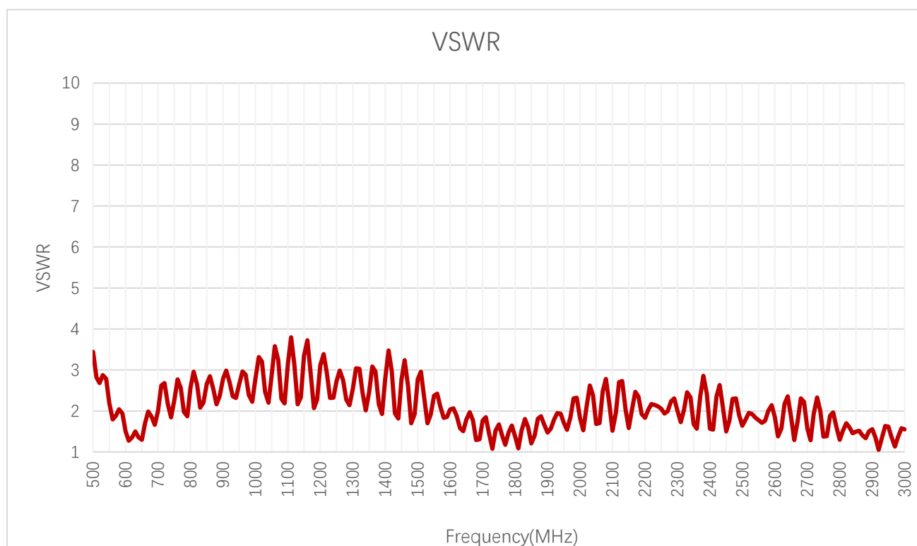
VSWR
