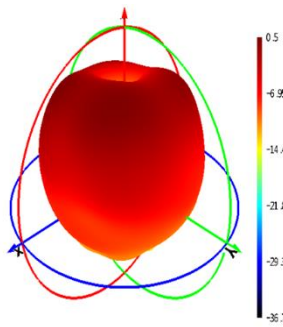
Phi=90
