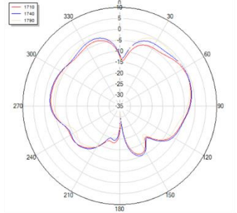
Phi=0
