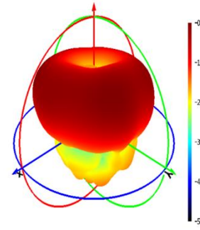
Phi=90
